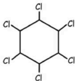
Benzene hexachloride (Gammaxene)
