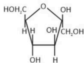
\beta -D-(-)-Fructofuranose
