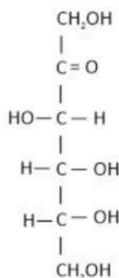
\alpha -D-(-)-Fructofuranose
