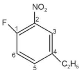
4-ethyl-1-fluoro-2-nitrobenzene
