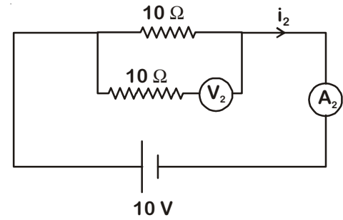
परिपथ 2
