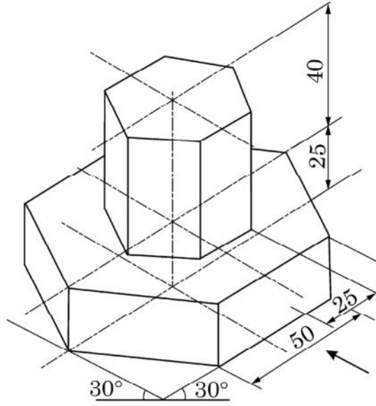
सममितीय प्रक्षेपण
